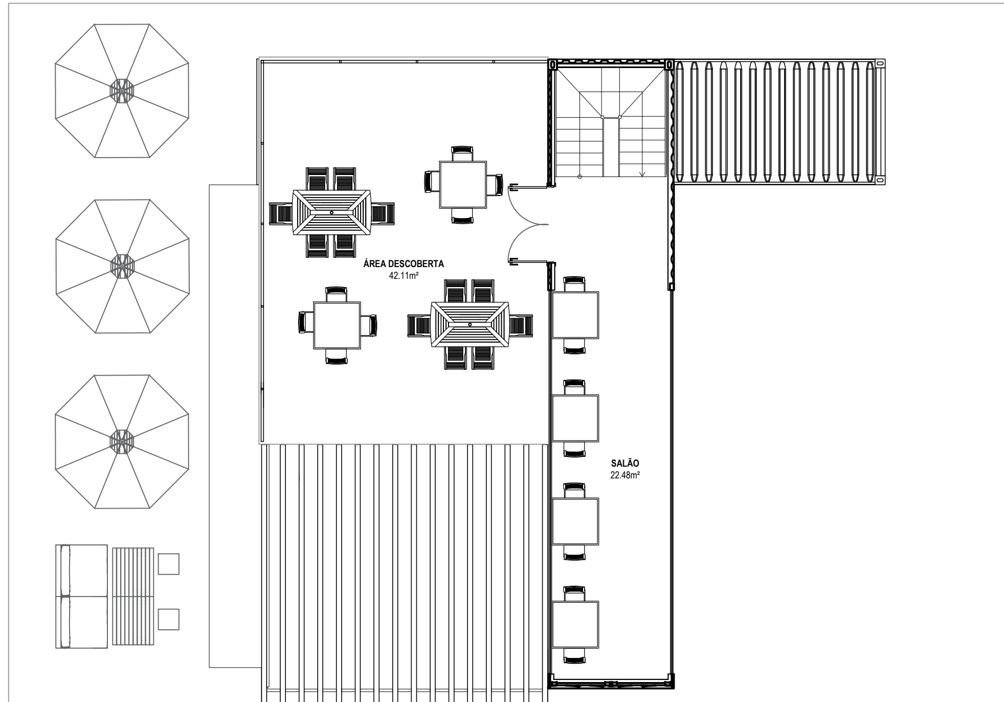
01 PLANTA BAIXA – 1º PAVIMENTO 1:75
