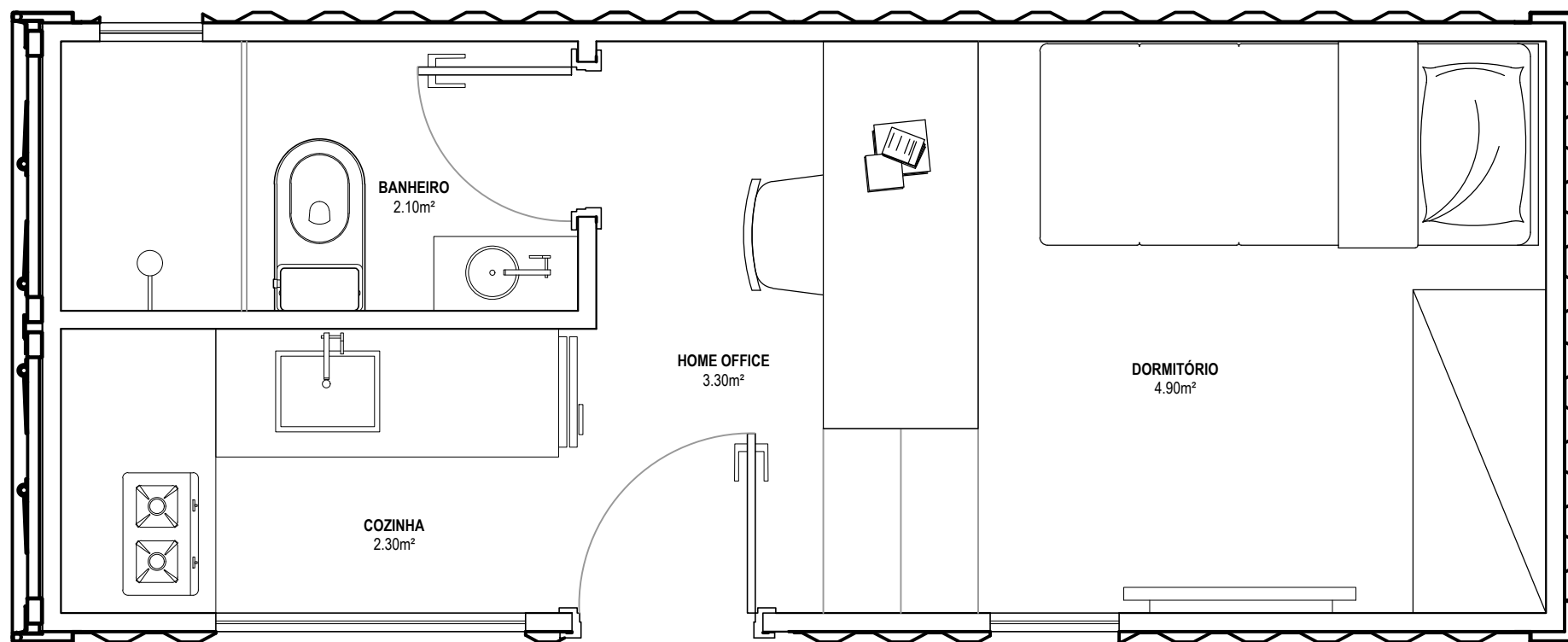
01 PLANTA BAIXA 1:25
